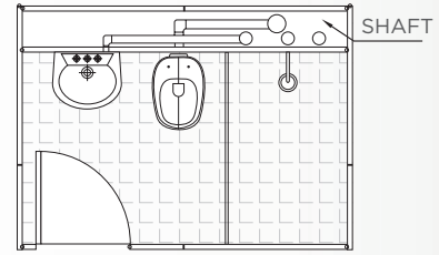
• Parede dupla com tubulação embutida
