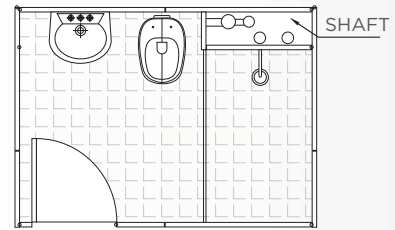
• Parede simples com tubulação aparente
